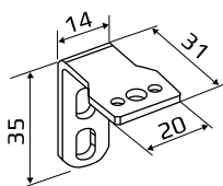
КРОНШТЕЙН СТЕНОВОЙ СТАНДАРТНЫЙ
