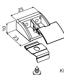
КРОНШТЕЙН СТЕНОВОЙ СТАНДАРТНЫЙ
