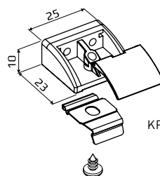
КРОНШТЕЙН СТЕНОВОЙ СТАНДАРТНЫЙ
