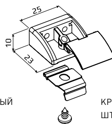
КРОНШТЕЙН СТЕНОВОЙ МАЛЫЙ
