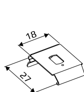
КРОНШТЕЙН ПОТОЛОЧНЫЙ
