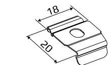
КРОНШТЕЙН ПЛОСКИЙ ПОТОЛОЧНЫЙ
