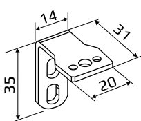
КРОНШТЕЙН СТЕНОВОЙ СТАНДАРТНЫЙ
