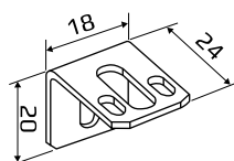
КРОНШТЕЙН СТЕНОВОЙ МАЛЫЙ
