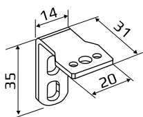
КРОНШТЕЙН СТЕНОВОЙ СТАНДАРТНЫЙ
