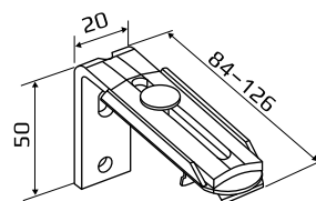
КРОНШТЕЙН СТЕНОВОЙ РЕГУЛИРУЕМЫЙ 60 — 108 ММ
