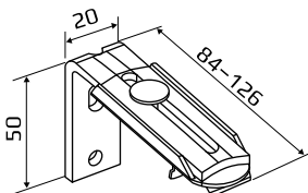
КРОНШТЕЙН СТЕНОВОЙ РЕГУЛИРУЕМЫЙ 60 — 108 ММ
