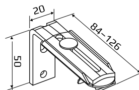
КРОНШТЕЙН СТЕНОВОЙ РЕГУЛИРУЕМЫЙ 60 — 108 ММ
