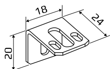
КРОНШТЕЙН СТЕНОВОЙ МАЛЫЙ
