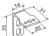
КРОНШТЕЙН СТЕНОВОЙ СТАНДАРТНЫЙ
