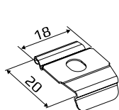
КРОНШТЕЙН ПЛОСКИЙ ПОТОЛОЧНЫЙ
