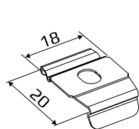
КРОНШТЕЙН ПЛОСКИЙ ПОТОЛОЧНЫЙ
