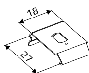
КРОНШТЕЙН ПОТОЛОЧНЫЙ
