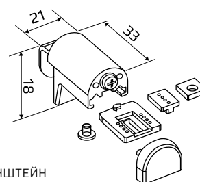
КРОНШТЕЙНЫ НА ШТАПИК
