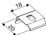
КРОНШТЕЙН ПОТОЛОЧНЫЙ СПЕЦИАЛЬНЫЙ
